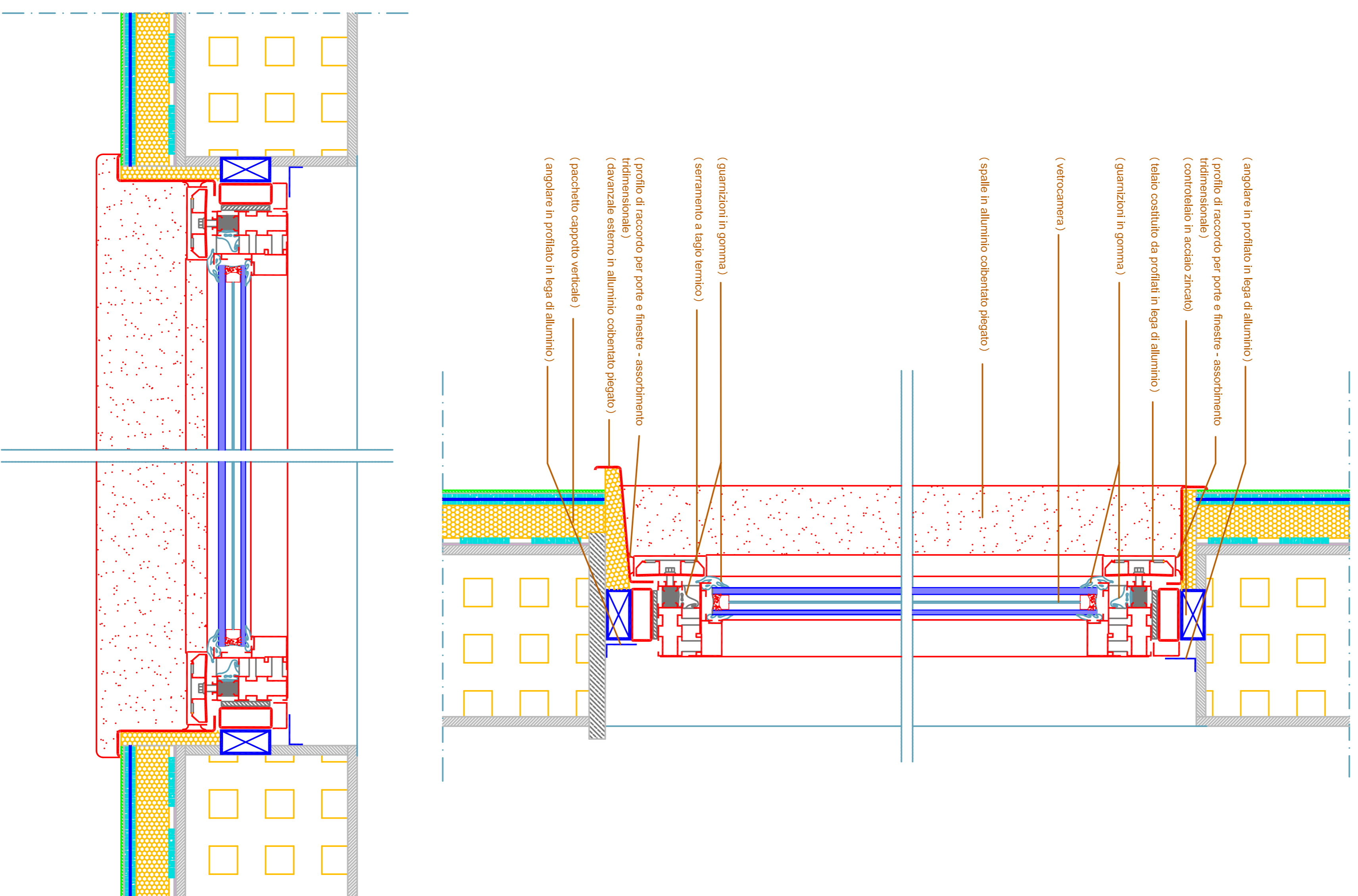
SISTEMA ISOLAMENTO TERMICO A CAPPOTTO PER ESTERNO.
